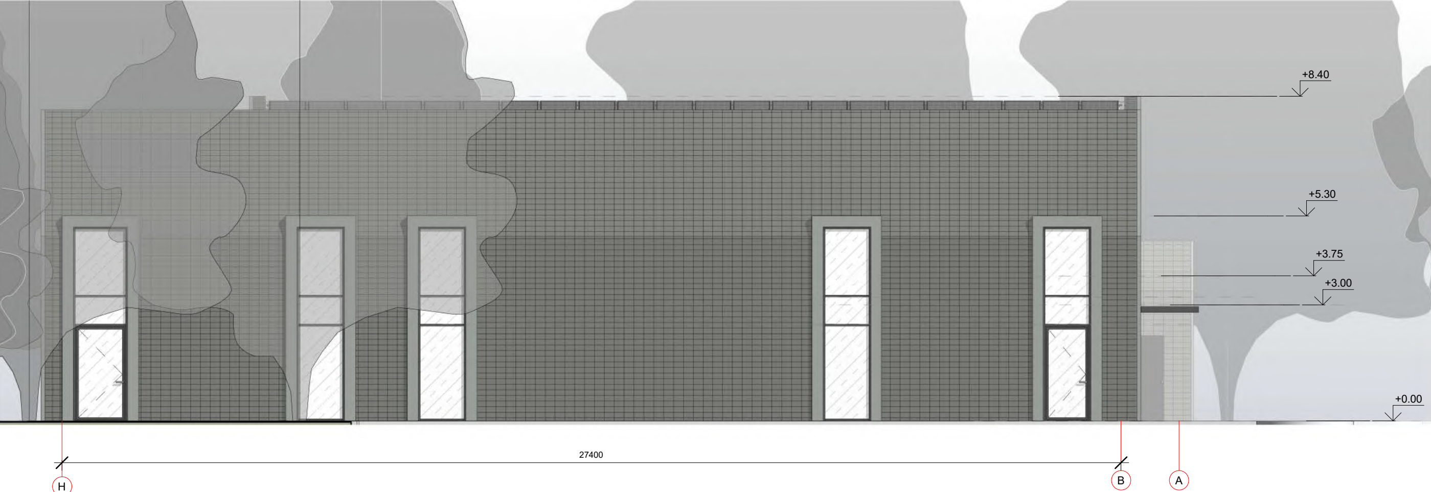
Fasadas E-A M 1 : 100
