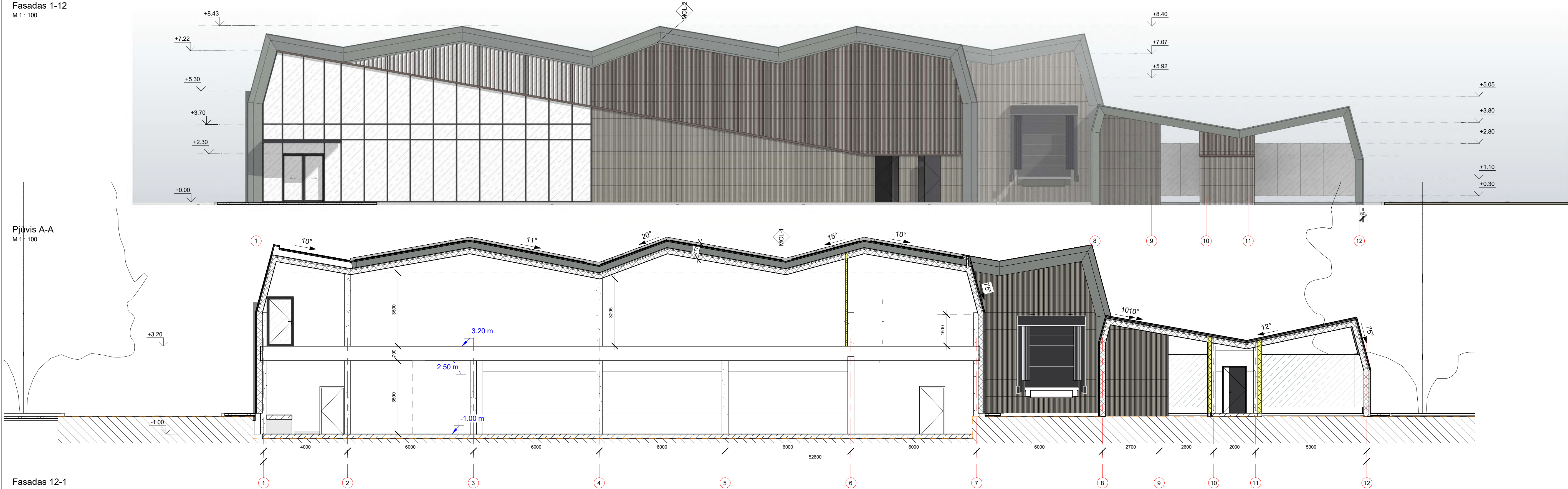
Fasadas 12-1 M 1 : 100
